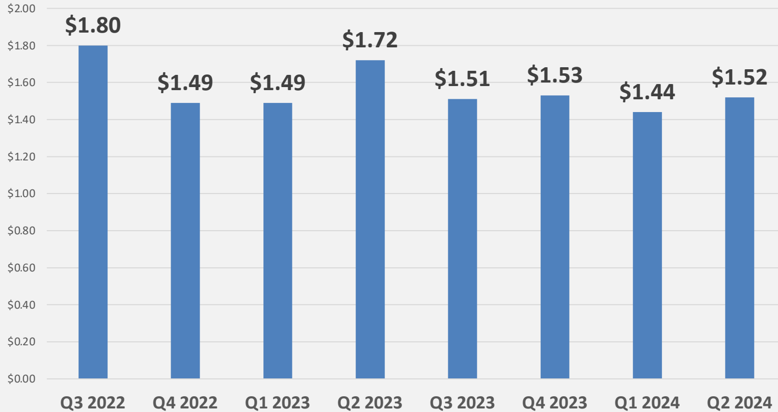
Chrome $/lb
